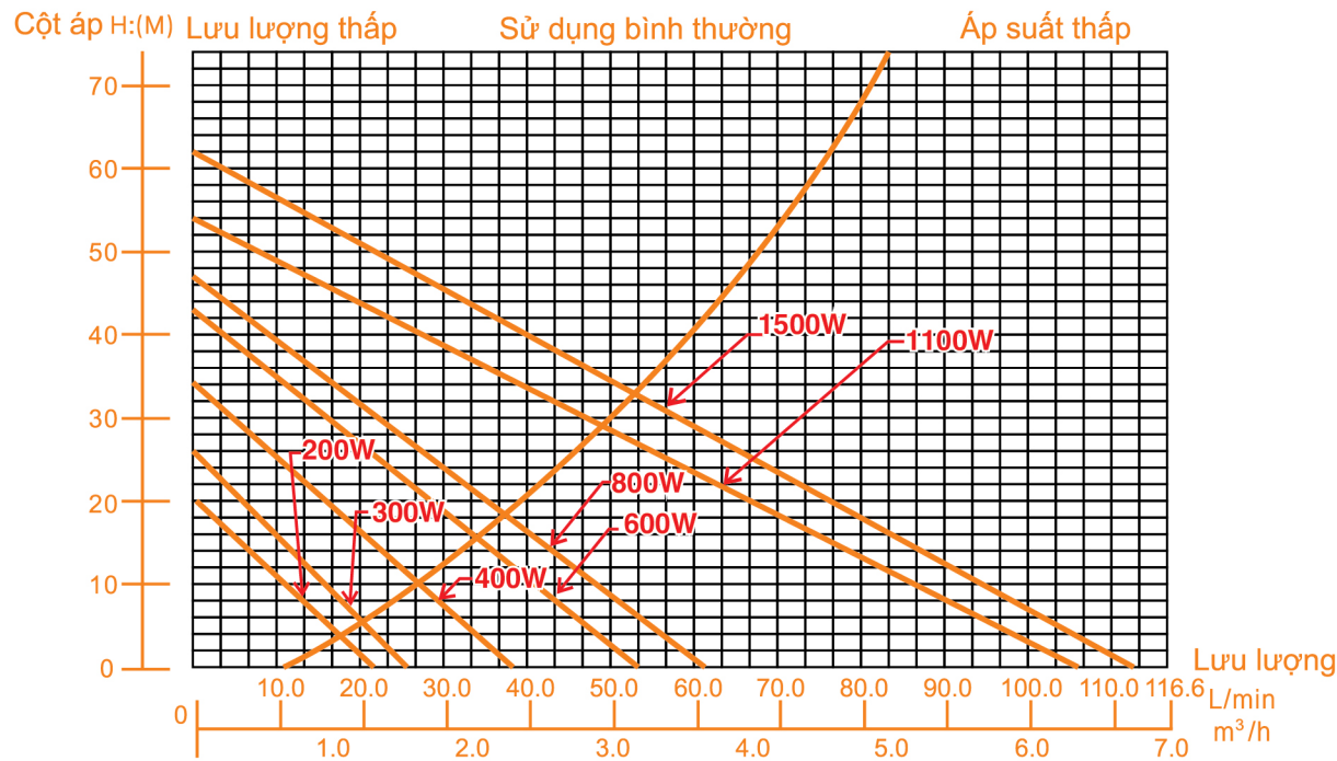
BIỂU ĐỒ HIỆU SUẤT CỦA MÁY
